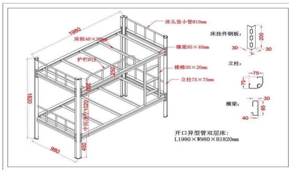
附件: 双层铁架床规格要求
